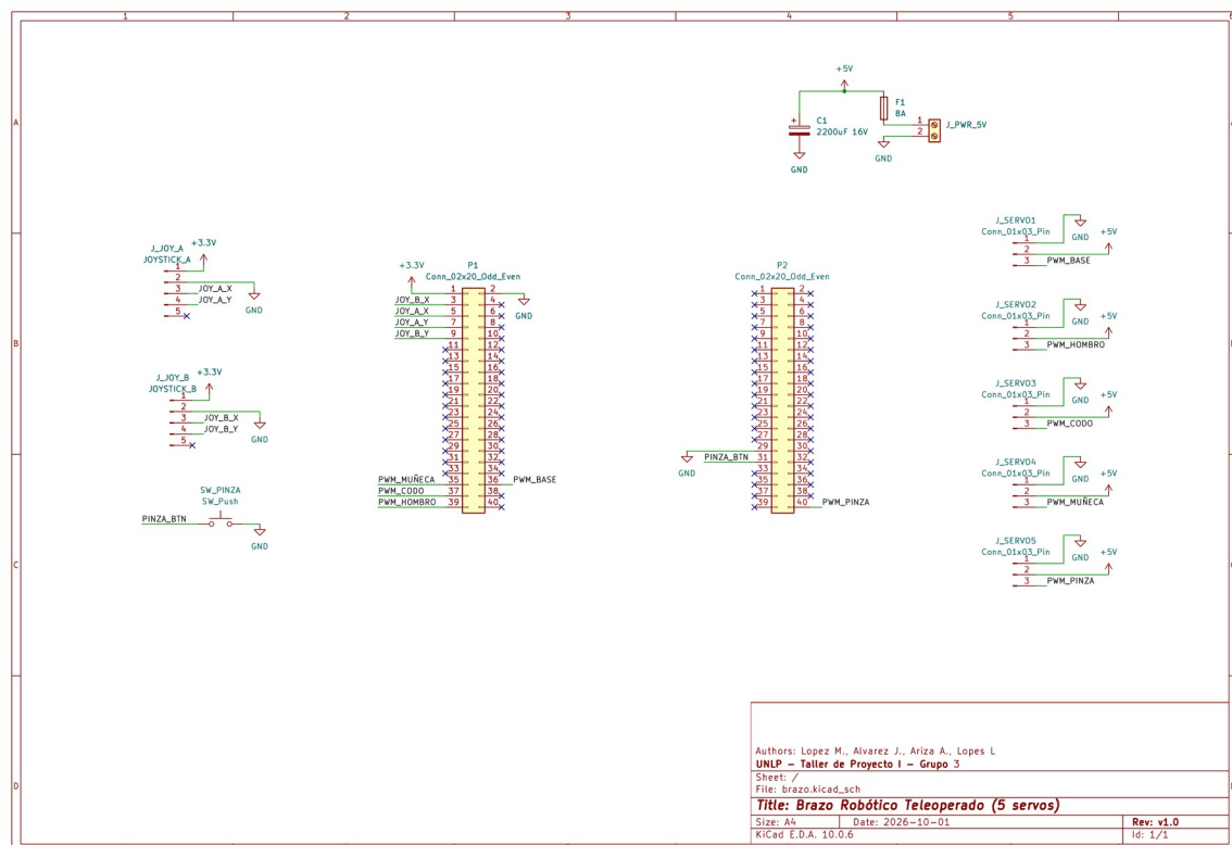
Figura A.1. Circuito esquemático general de conexiones de la EDU-CIAA-NXP y periféricos.
