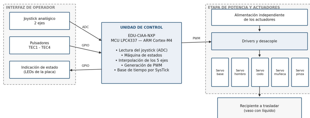
Fig. 1: Diagrama en bloques del sistema a desarrollar.
