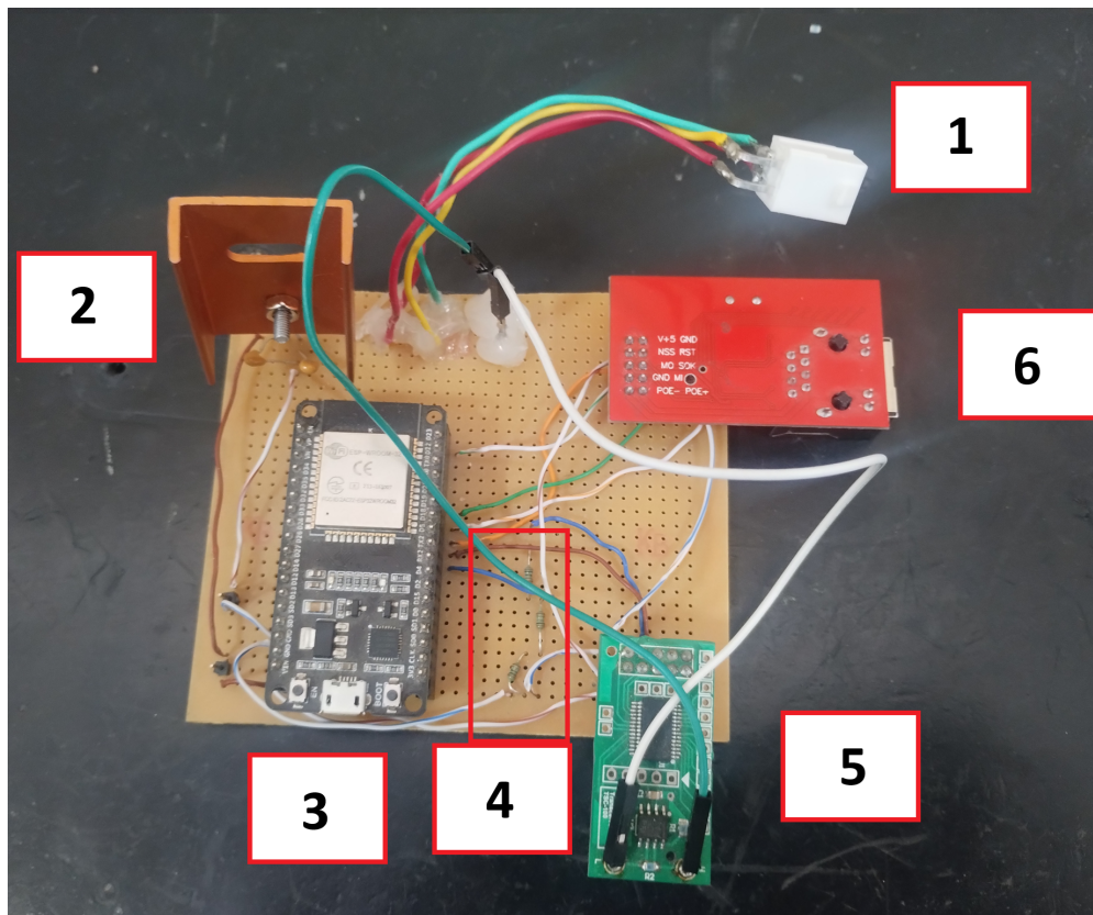
FIGURA 3.5. Prototipo experimental del equipo.
