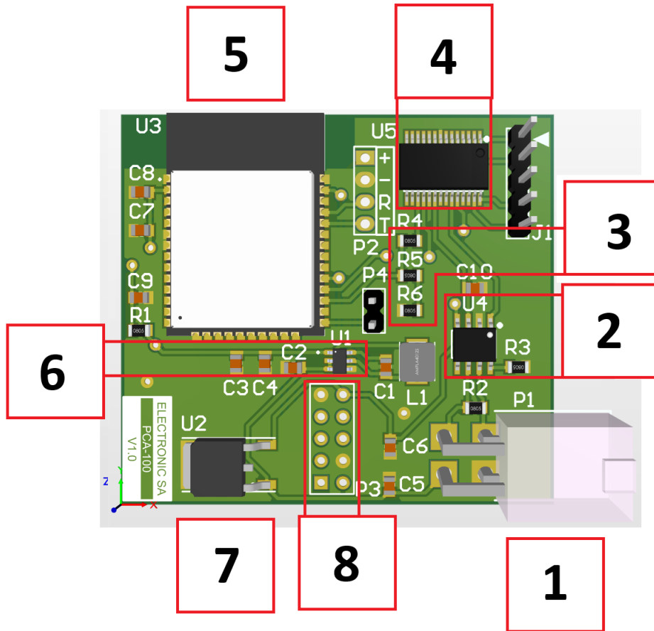
FIGURA 3.6. Diseño final para PCB del equipo.
