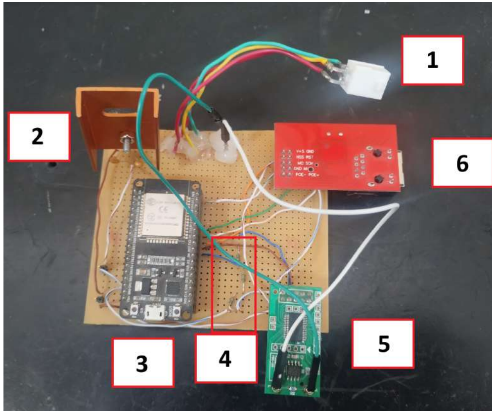
FIGURA 4.6. Prototipo experimental del equipo.
