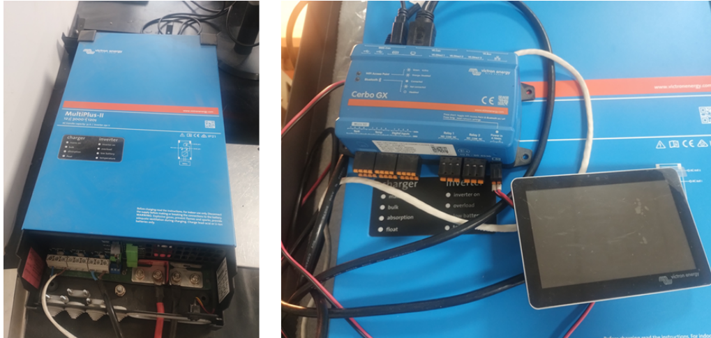
FIGURA 4.13. Equipo Victron MultiPlus-II y módulo Cerbo GX.
