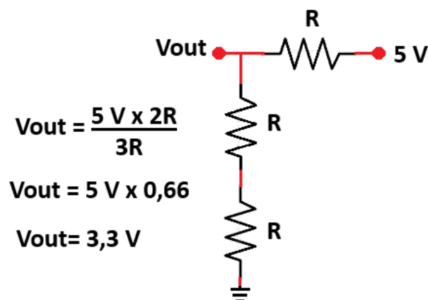
FIGURA 3.4. Diseño de divisor resistivo para adaptación UART.
