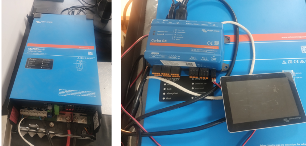
FIGURA 4.9. Equipo Victron MultiPlus-II y módulo Cerbo GX.
