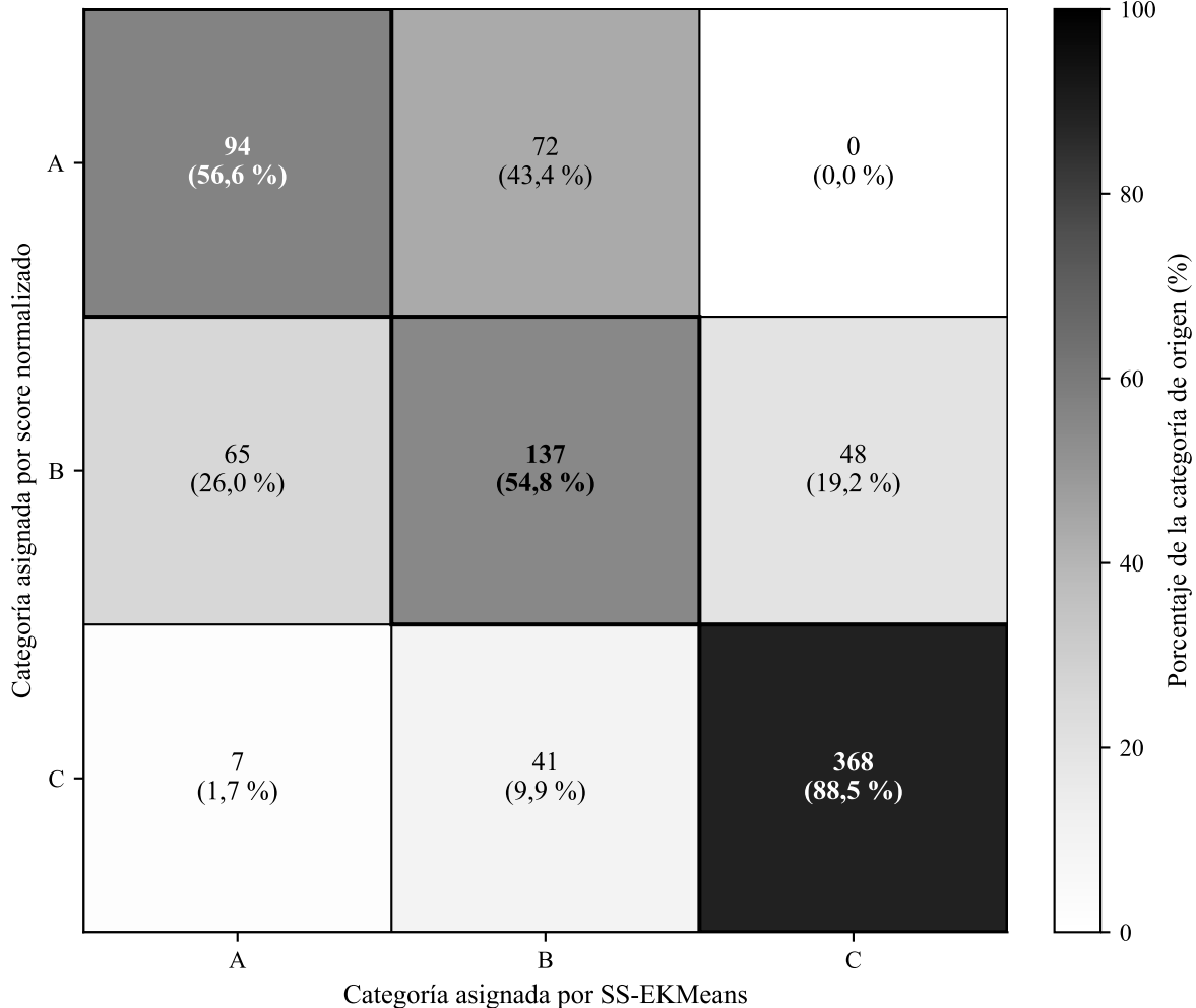
Matriz de transición entre métodos Coincidencia exacta: 72,00 % · ARI: 0,4678
