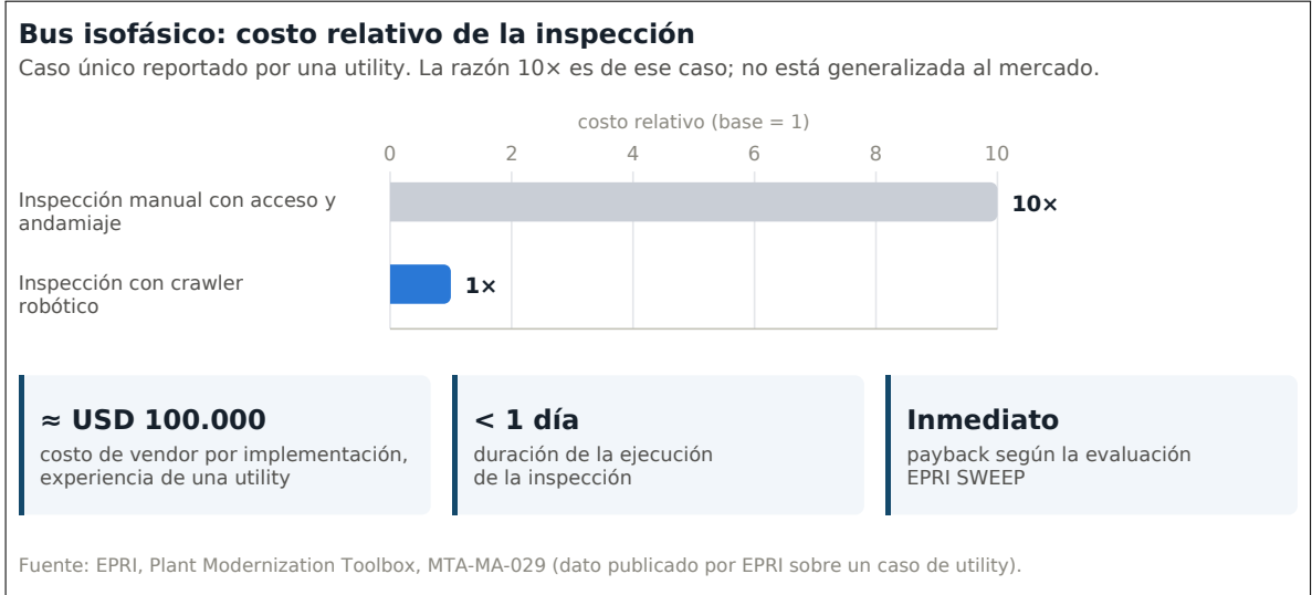
Figura 7 — Costo relativo de la inspección de bus isofásico e indicadores del caso reportado. EPRI, Plant Modernization Toolbox, MTA-MA-029.
