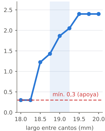
Juego a la placa de cámara peor caso vs. largo del flex
