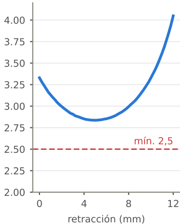
R interior vs. retracción (L = 19,0, cotas nominales)
