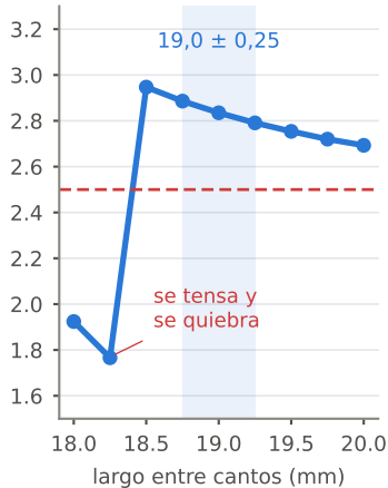
R interior peor caso vs. largo del flex
