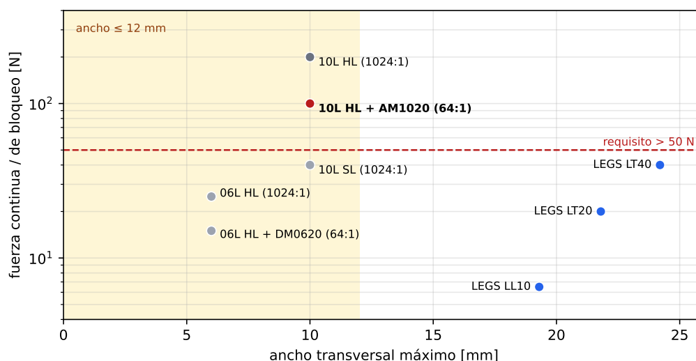
Figura 5: Fuerza continua (FAULHABER) o de bloqueo (PiezoMotor) frente al ancho transversal máximo, según las hojas de datos. Solo el 10L HL cae en la zona de ≤12 mm y >50 N.
