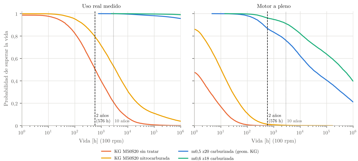
Figura 9: Probabilidad de que el par supere una vida dada. Línea de trazos: objetivo de 2 años (576 h).
