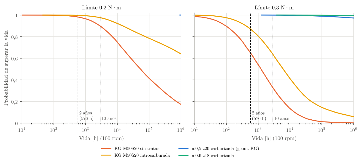
Figura 11: Probabilidad de superar una vida dada con cada límite de torque.
