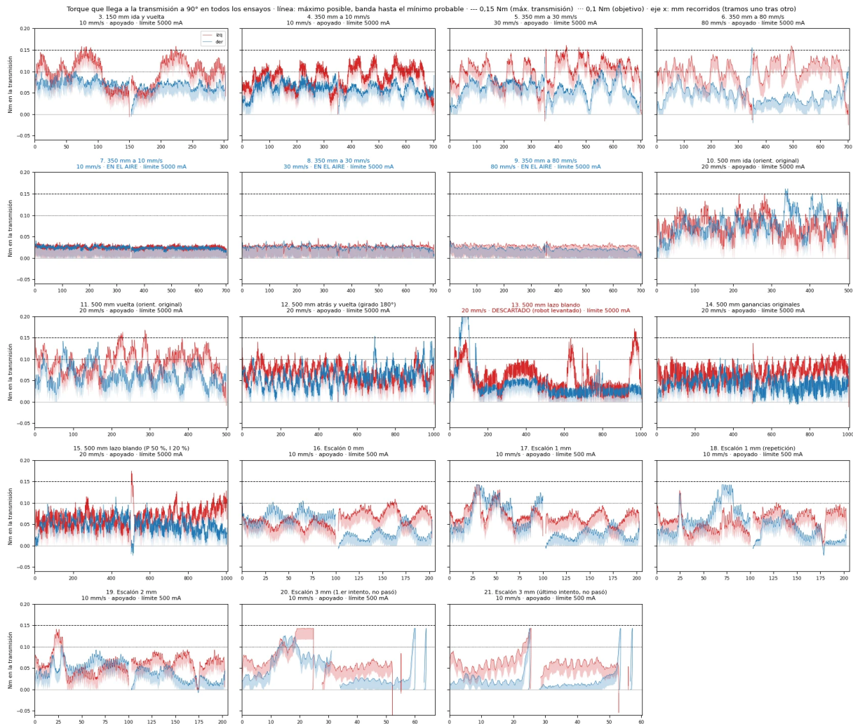
Figura 10: Torque que llega a la transmisión a 90° en los ensayos 3 a 21 (izquierda en rojo, derecha en azul; línea: máximo posible; banda: hasta el mínimo probable). Fuente: ensayos del robot, provistos por el usuario.
