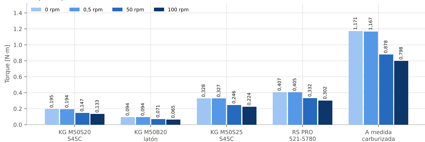
Torque de pico admisible (10 s, ocasional)
