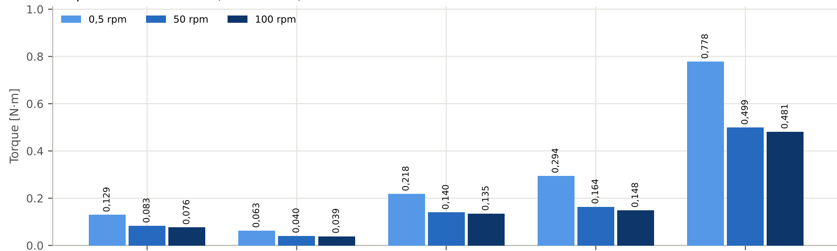
Torque de pico admisible (10 s, ocasional)
