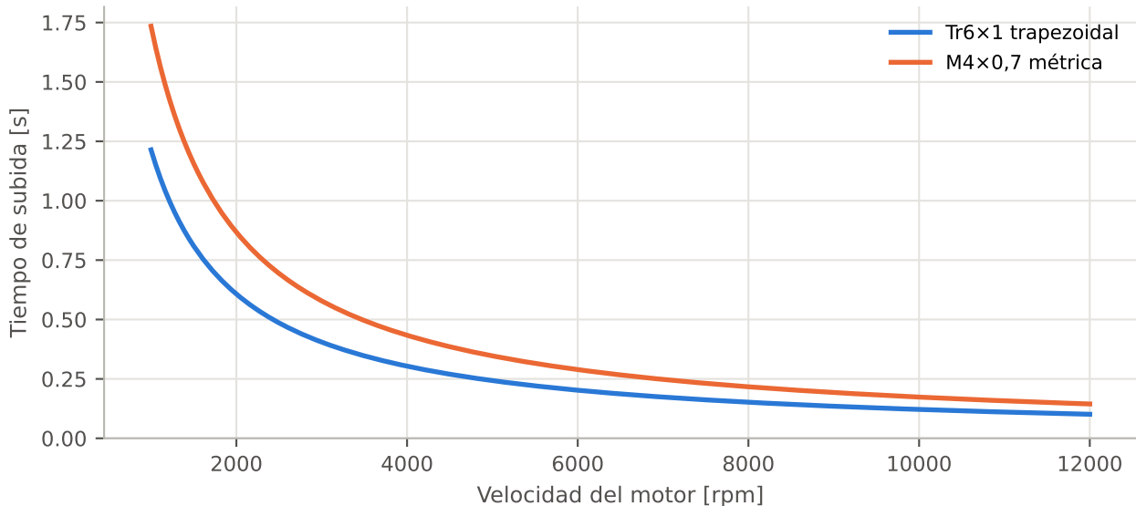
Tiempo de subida completa (carrera de la tuerca 20.2 mm), sin reductor
