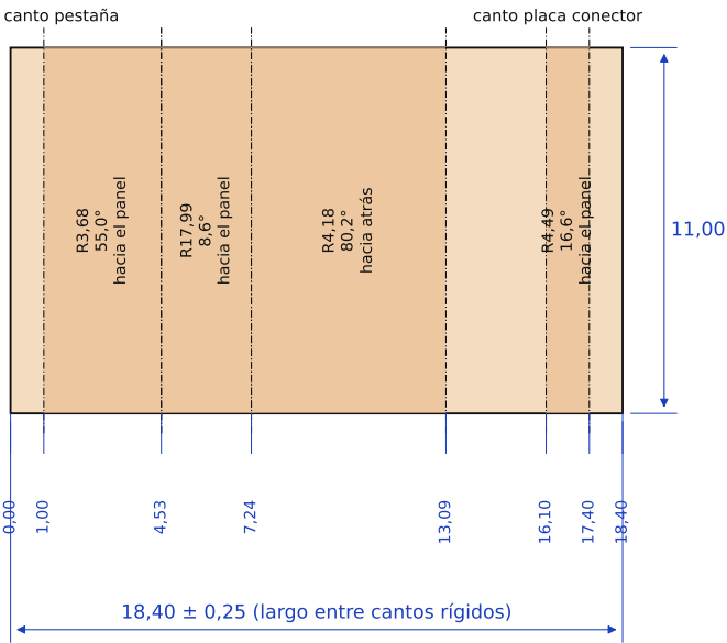
DESARROLLO DE LA TIRA (plano) — ESCALA 4:1
