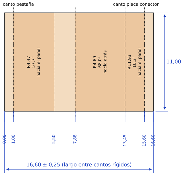
DESARROLLO DE LA TIRA (plano) — ESCALA 4:1
