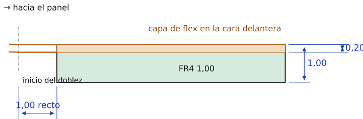
DETALLE A — SALIDA EN LA PLACA DEL CONECTOR — ESCALA 10:1
