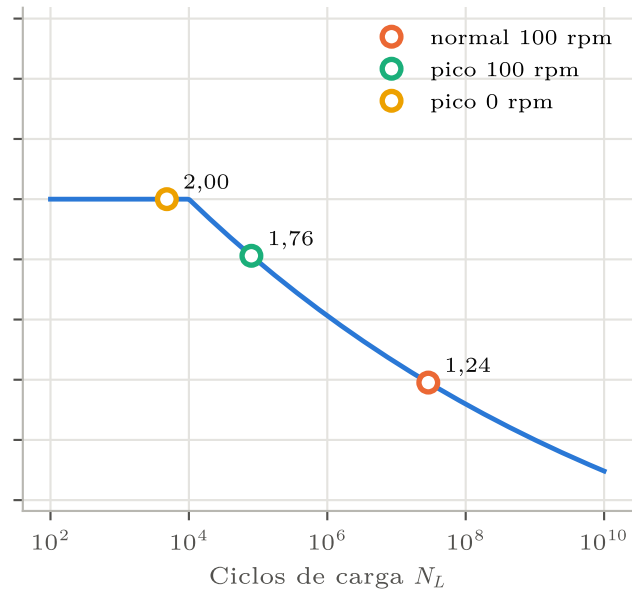
Picado Z_{NT} (Fig. 15-8)
