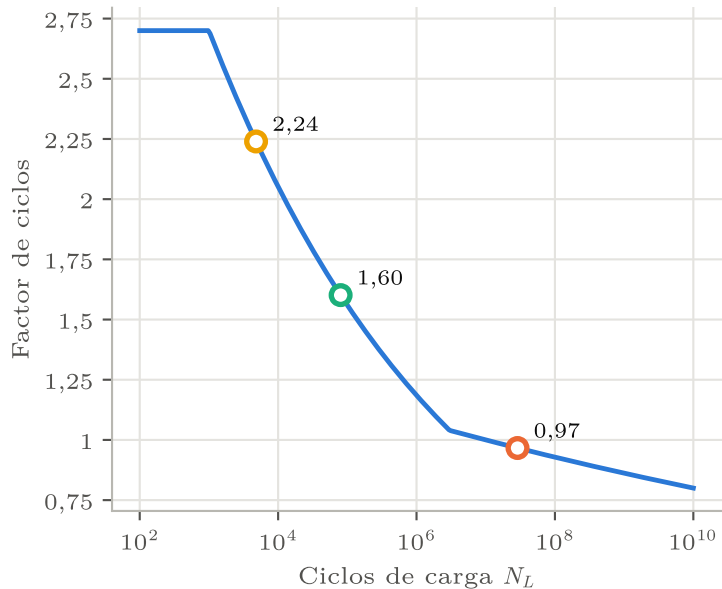
Flexión Y_{NT} (Fig. 15-9)
