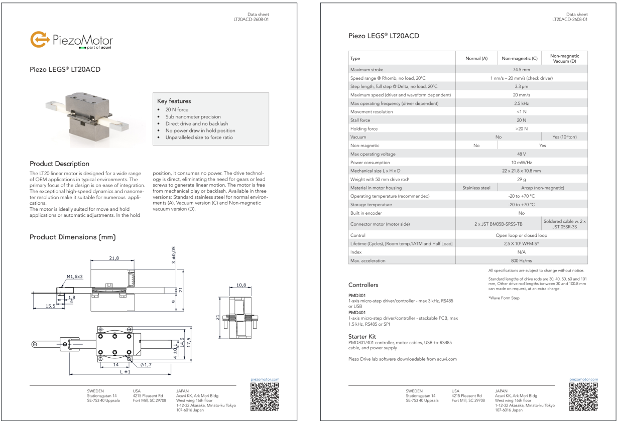
Figura 7: Hoja PiezoMotor LT20ACD: 20 N de bloqueo en 22×21,8×10,8 mm.
