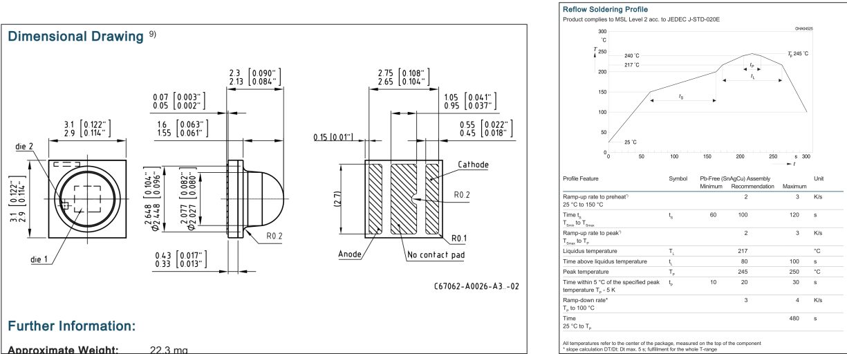
Figura 9: Plano dimensional (p. 16) y perfil de reflow, MSL 2 (p. 18).
