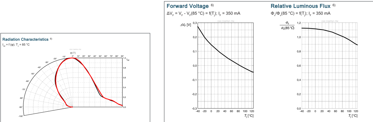
Figura 8: Diagrama de radiación (p. 12) y variación de V_F y flujo con T_j (p. 14).
