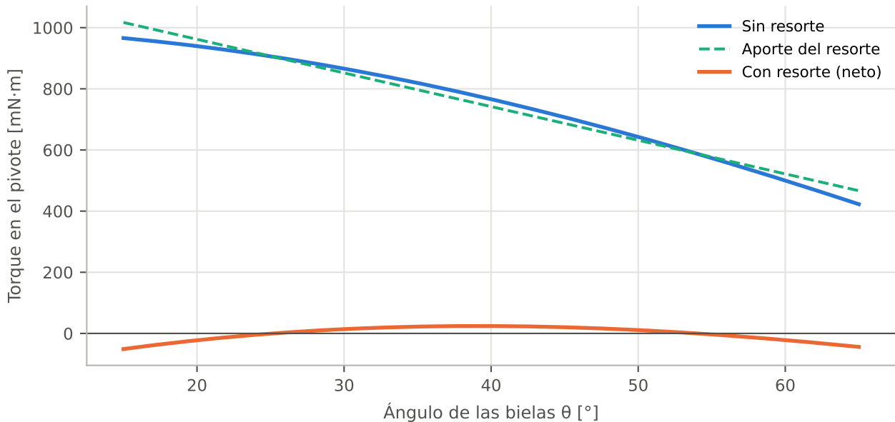
Compensación con resorte de torsión ( k \approx 11.0 \text{ mN}\cdot\text{m}/^\circ )
