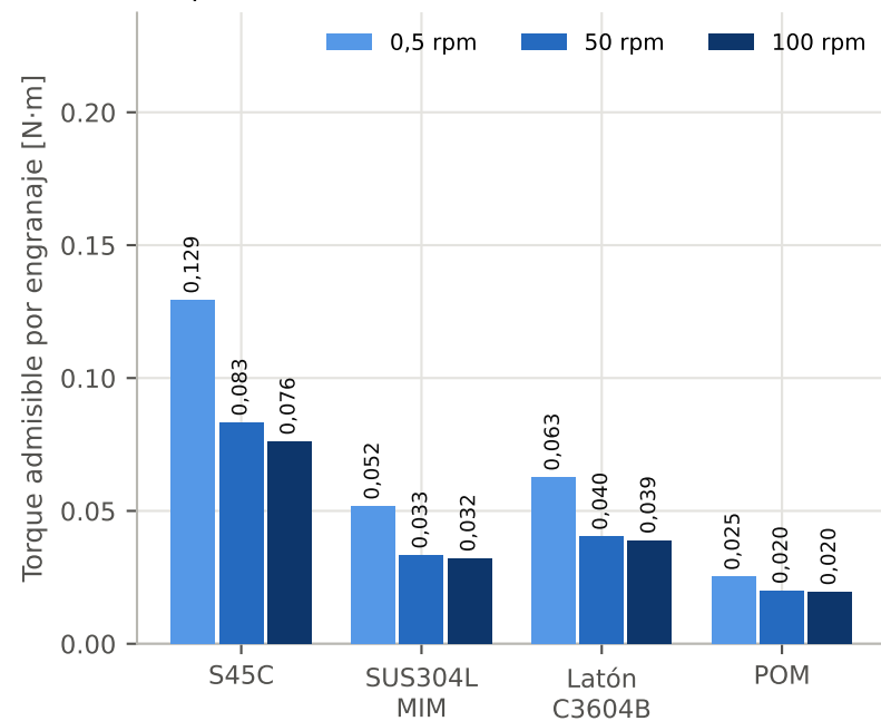
Torque normal (toda la vida)
