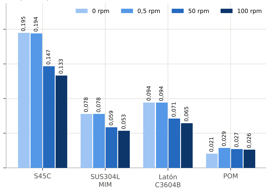
Torque de pico (10 s, ocasional)
