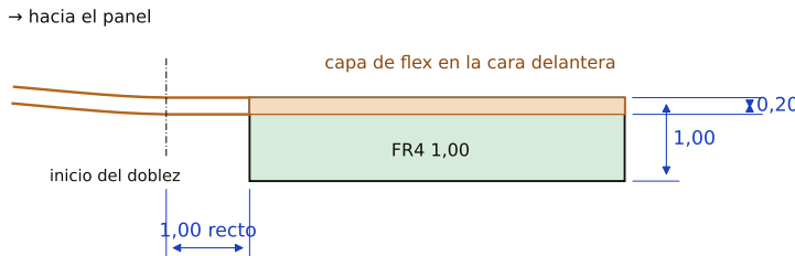
DETALLE A — SALIDA EN LA PLACA DEL CONECTOR — ESCALA 10:1
