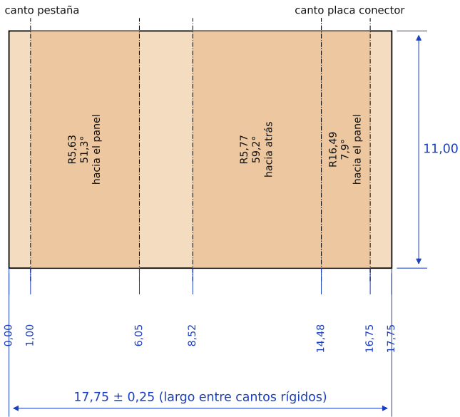
DESARROLLO DE LA TIRA (plano) — ESCALA 4:1
