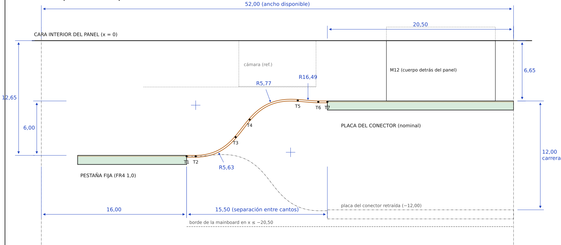
PLANTA (vista de arriba) — ESCALA 4:1
