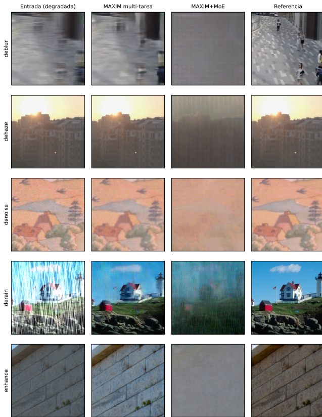
FIG. 3. Comparación cualitativa sobre muestras de validación de distintas tareas. De izquierda a derecha: entrada degradada, MAXIM multi-tarea, MAXIM+MoE e imagen de referencia. La figura se genera con el script eval_metrics.py a partir de los checkpoints guardados.
