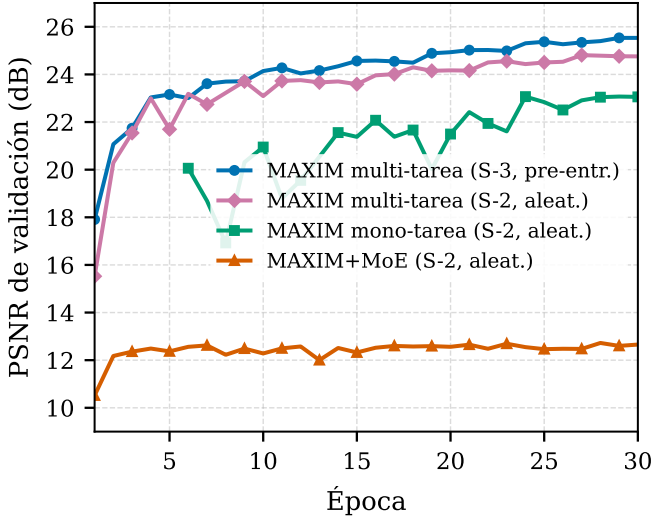
FIG. 1. Evolución de la PSNR de validación durante el entrenamiento, para un presupuesto común de 30 épocas. Las tres versiones de MAXIM sin MoE —multi-tarea pre-entrenada (S-3), multi-tarea desde cero (S-2) y mono-tarea (S-2)— mejoran de forma sostenida y se agrupan por encima de 23 dB, mientras que la variante MAXIM+MoE se estanca tempranamente en torno a 12,7 dB. La comparación más justa es entre MAXIM+MoE y la multi-tarea desde cero, que comparten escala e inicialización. La curva mono-tarea comienza en la época 6 por el rango disponible en el registro de entrenamiento.
