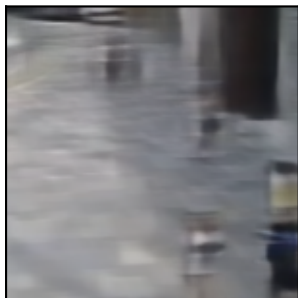
MAXIM multi-tarea
