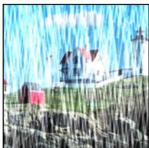
derain
