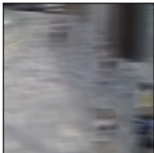
Entrada (degradada)
