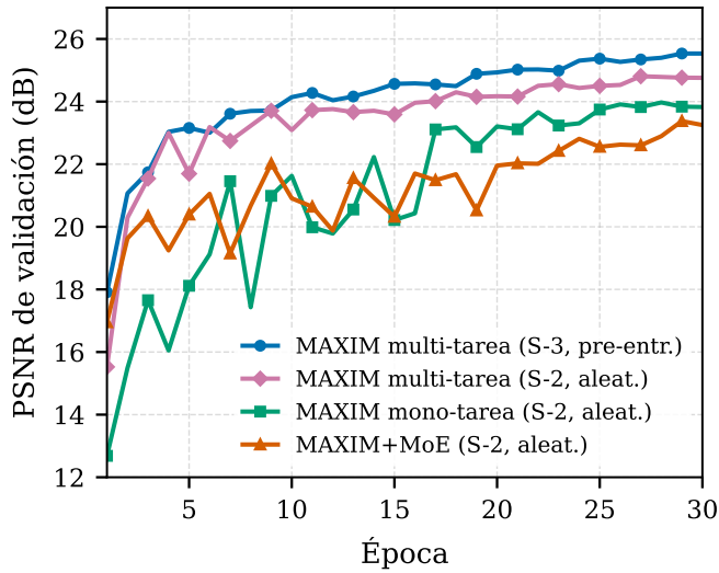
FIG. 4. Evolución de la PSNR de validación durante el entrenamiento, para un presupuesto común de 30 épocas. Las dos versiones multi-tarea de MAXIM sin MoE convergen a 24,8–25,5 dB, y la mono-tarea alcanza 24,0 dB sobre su única tarea (realce). La variante MAXIM+MoE converge a 23,4 dB, aproximadamente 1,4 dB por debajo de la multi-tarea desde cero, con la que comparte escala (S-2), inicialización aleatoria y datos, y que constituye por ello la comparación más justa.
