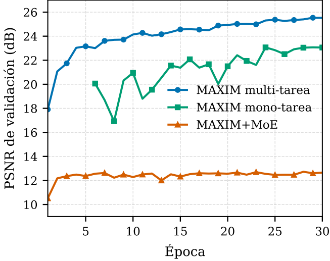
FIG. 1. Evolución de la PSNR de validación durante el entrenamiento, para un presupuesto común de 30 épocas. Las dos versiones de MAXIM sin MoE mejoran de forma sostenida, mientras que la variante MAXIM+MoE se estanca tempranamente muy por debajo de ambas. La curva mono-tarea comienza en la época 6 por el rango disponible en el registro de entrenamiento.
