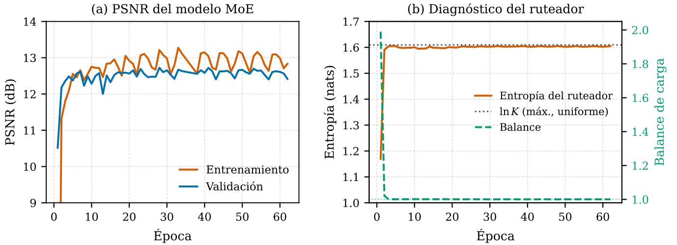
FIG. 2. Diagnóstico de la variante MAXIM+MoE a lo largo de 62 épocas. (a) La PSNR de entrenamiento y validación se estancan en torno a 12,5–13 dB. (b) La entropía del ruteador (naranja) satura en su máximo \ln K (línea punteada gris) y el balance de carga (verde) cae a su mínimo 1,0; el ruteo colapsa a un régimen uniforme y no especializado.
