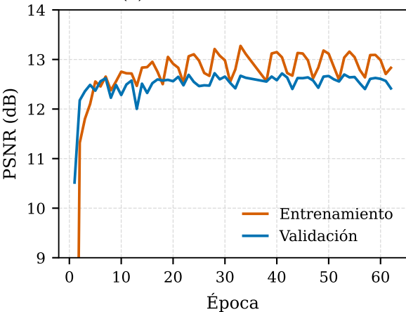
(a) PSNR del modelo MoE
