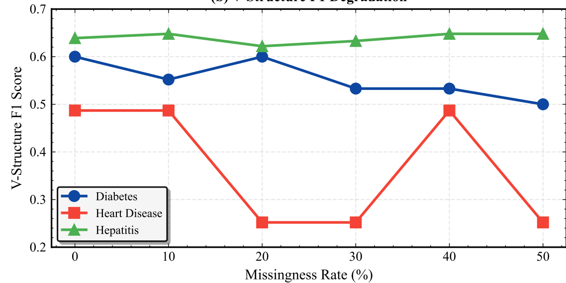
(b) V-Structure F1 Degradation
