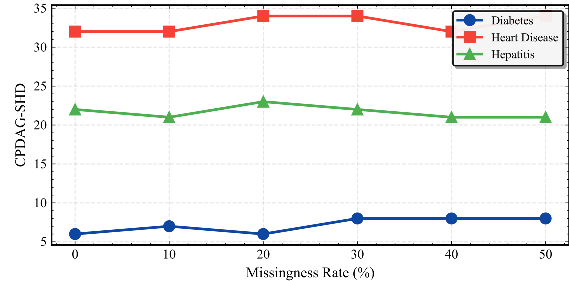
(d) CPDAG-SHD Increase
