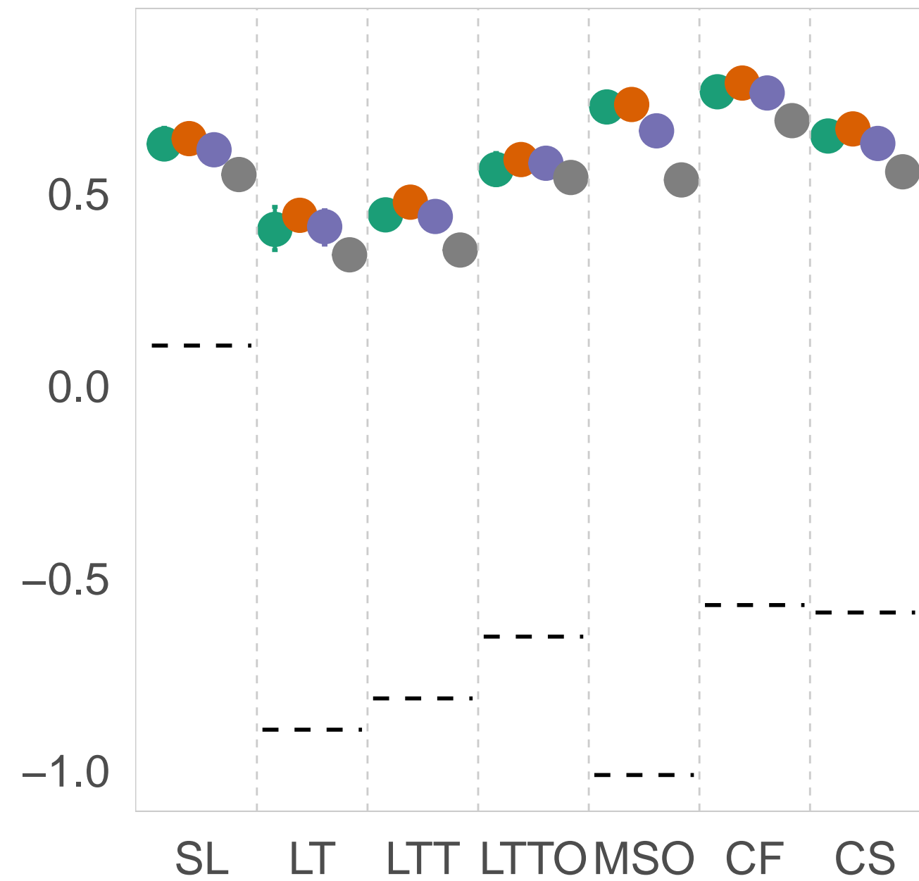
FFN
