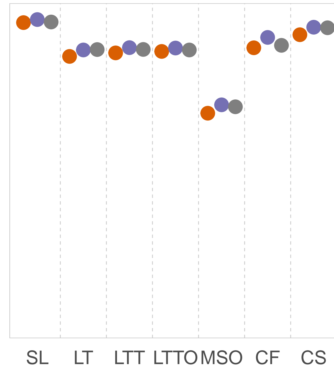
GRU
