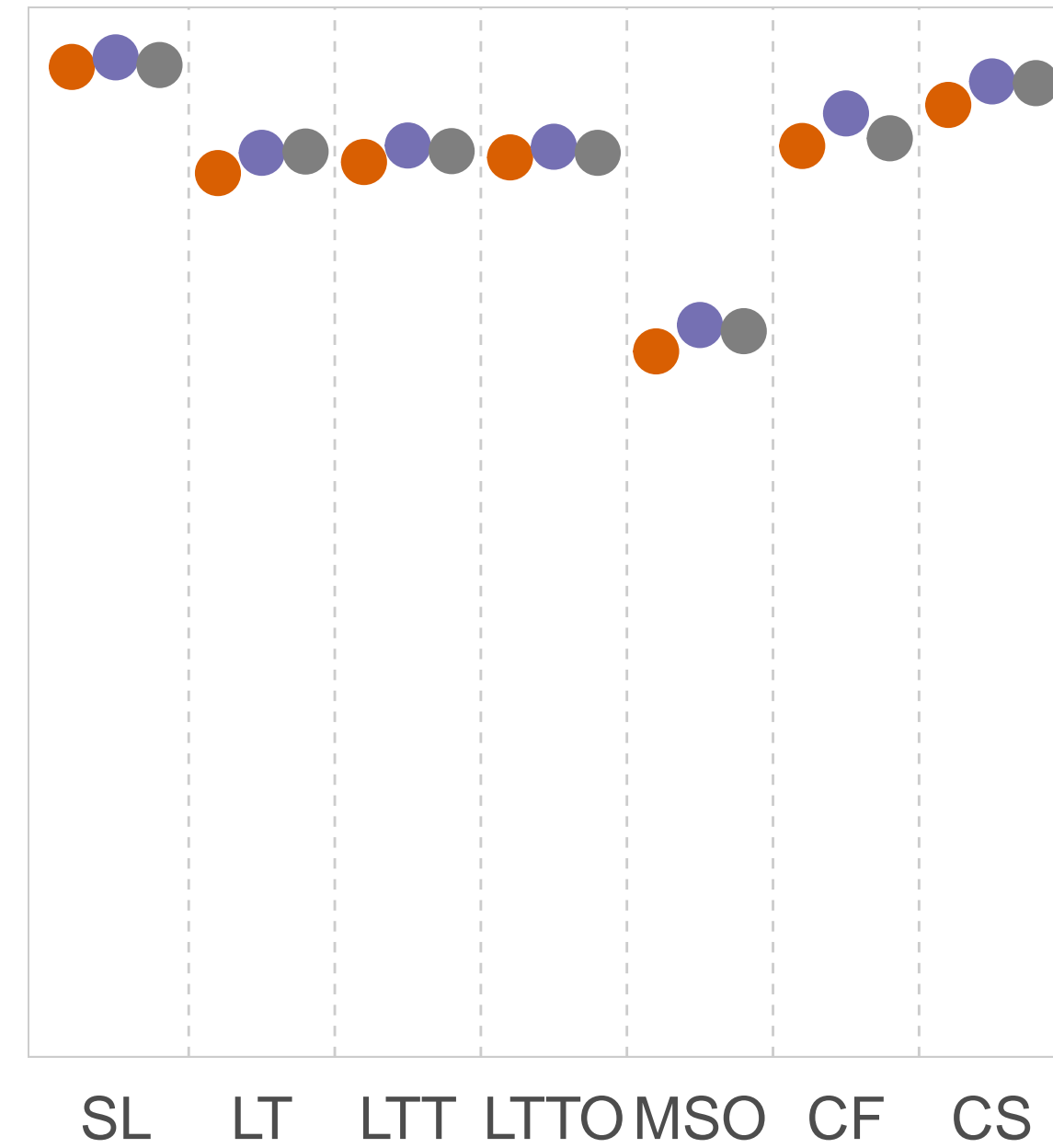
GRU
