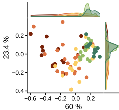
Foraminifera
