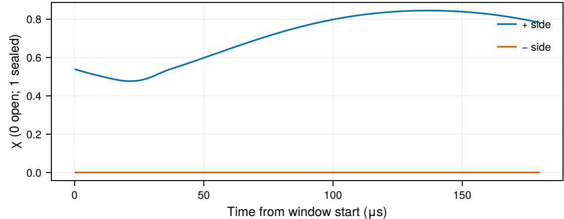
Hydraulic sealing parameter
