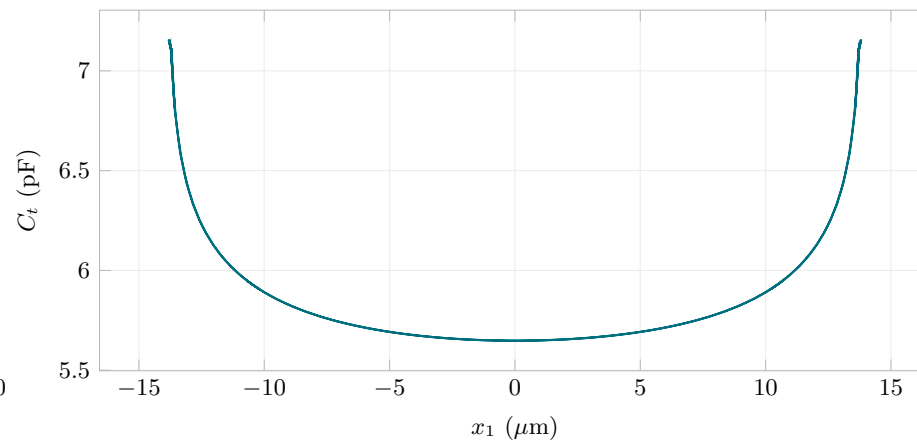
(d) Capacitance along the mechanical cycle
