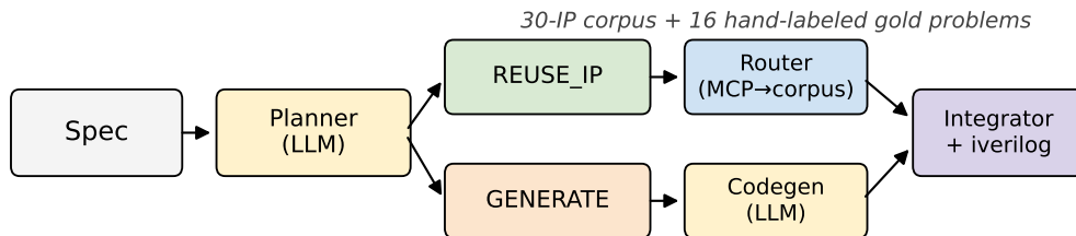
(a) Per-LLM evaluation pipeline
