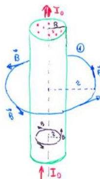
Figure 125: Campo Magnetico di un Filo Rettilineo
