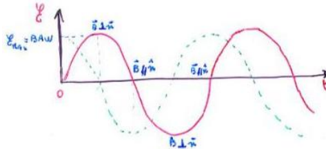
Figure 170: Tratteggiato è l'andamento di \phi_B
