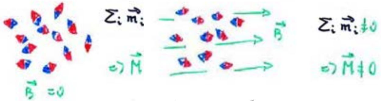
(b) In Presenza Di Un Campo \vec{B} I Dipoli Rustano Etendono Ad Aggirarsi Con Il Campo \vec{B}
