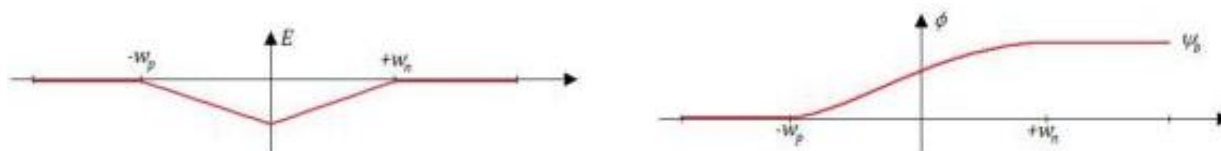
(a) Campo elettrico in un diodo a giunzione pn
