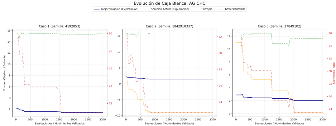
Figura 3: Evolución de Caja Blanca para el algoritmo CHC. Las caídas escalonadas en la Función Objetivo representan las fases de convergencia, seguidas de reinicios poblacionales que reinyectan diversidad estructural al sistema.
