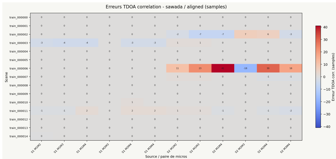
FIGURE 6 – Analyse quantitative des TDOA estimates par correlation sur les sources separees en présence de bruit.
