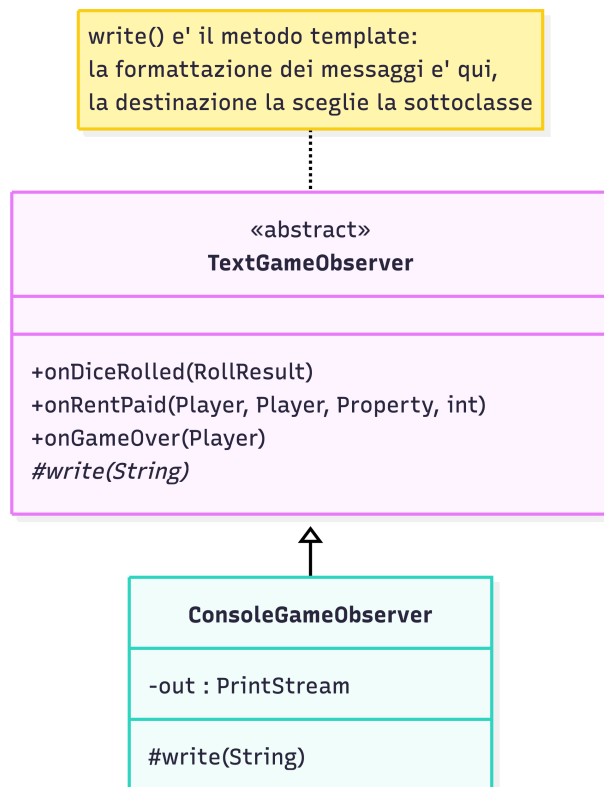
Figura 2.4: Template Method: TextGameObserver definisce il contenuto dei messaggi, mentre la sottoclasse ConsoleGameObserver decide solo dove scriverli, implementando il metodo template write .
