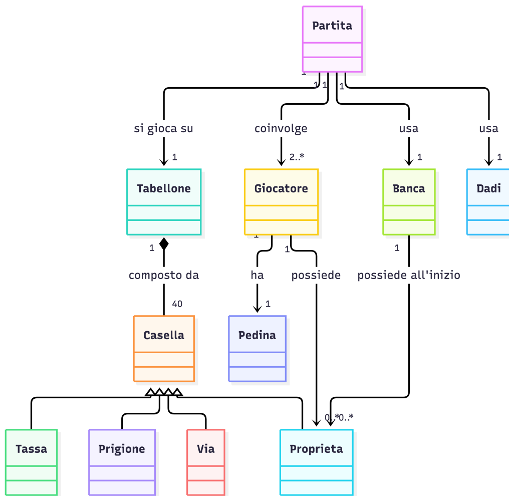
Figura 1.1: Schema del modello del dominio: le entità principali del gioco e i loro rapporti.
