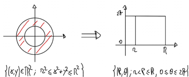
Figura 2.58: Trasformazione nel piano (\rho, \theta) .
