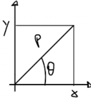
Figura 2.53: Rappresentazione di \vec{F}(\rho, \theta) = (F_1(\rho, \theta), F_2(\rho, \theta)) = (\rho \cos \theta, \rho \sin \theta) .
