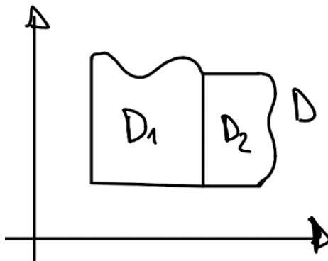
Figura 2.50: Esempio di dominio generale scomposto in domini semplici.
