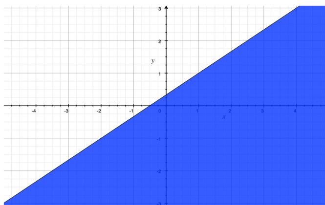
Figura 2.27: Sottografico di 2x - 3y + 1 = 0 .
