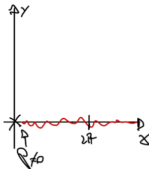
Figura 2.54: Dominio ( A ) dell'applicazione vettoriale \vec{F}(\rho, \theta) = (F_1(\rho, \theta), F_2(\rho, \theta)) = (\rho \cos \theta, \rho \sin \theta) . È esclusa la semiretta y = 0, x > 0 perché è un aperto e non sono considerati 0 e 2\pi .
