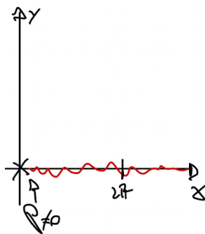
Figura 2.54: Dominio ( A ) dell'applicazione vettoriale \vec{F}(\rho, \theta) = (F_1(\rho, \theta), F_2(\rho, \theta)) = (\rho \cos \theta, \rho \sin \theta) . È esclusa la semiretta y = 0, x > 0 perché è un aperto e non sono considerati 0 e 2\pi .
