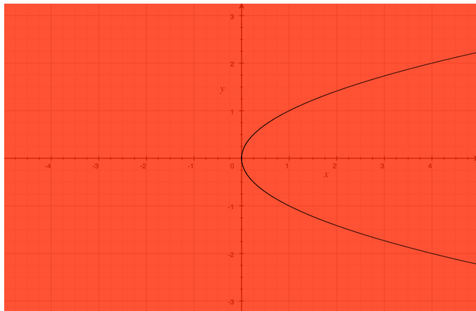
Figura 2.5: Grafico di A_2 = \{(x, y) \in \mathbb{R}^2 : x \neq y^2\} .
