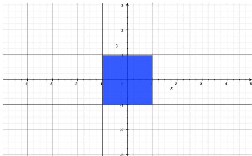
Figura 2.30: Dominio E = \{(x, y) \in \mathbb{R}^2 \mid 1 - x^2 \geq 0, 1 - y^2 \geq 0\} di z = \sqrt{1 - x^2} + \sqrt{1 - y^2} .
