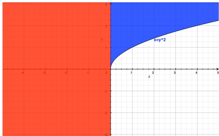
Figura 2.31: Dominio (in blu) E = \{(x, y) \in \mathbb{R}^2 \mid y > \sqrt{x}, x \geq 0\} di z = \frac{1}{\sqrt{y-\sqrt{x}}} .
