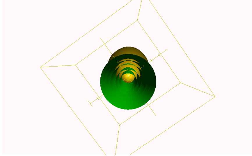
Figura 2.21: Grafico di z = f(x, y) = x^2 + y^2 intersecato con E_k .
