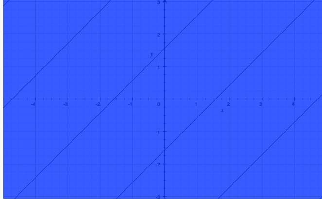
Figura 2.8: Grafico di A = \{(x, y) \in \mathbb{R}^2; (x, y) \neq (0, 0), y \neq x + \frac{\pi}{2} + k\pi, \forall k \in \mathbb{Z}\} .
