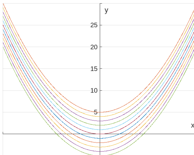
Figura 2.16: Grafico di z = k = x^2 - y , con k \in [-5, 5] \subset \mathbb{N} (nella realtà è \forall k \in \mathbb{R} ).
