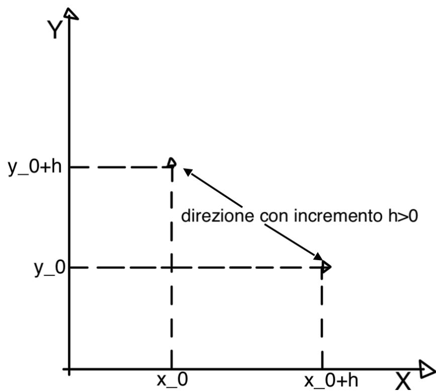
Figura 2.32: Rappresentazione delle direzioni con incremento h > 0 .
