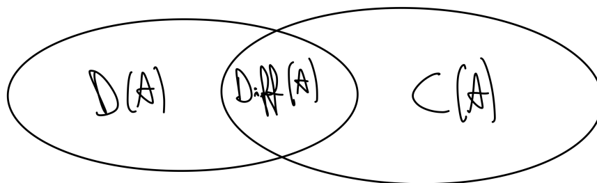
Figura 2.36: Insiemi di funzioni.
