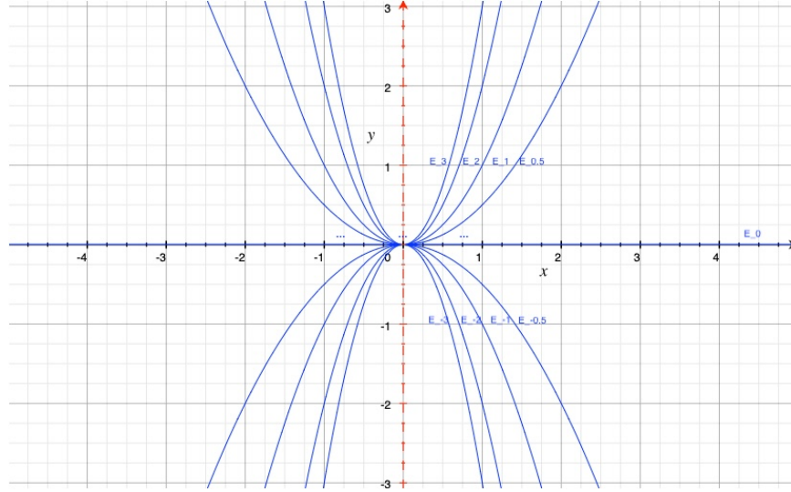
Figura 2.23: Grafico di E_k = \{(x, y) \in E \mid \frac{y}{x^2} = k\} (asse y escluso).
