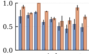
(d) F1
