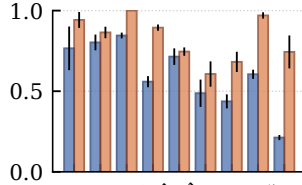
(e) AUC
